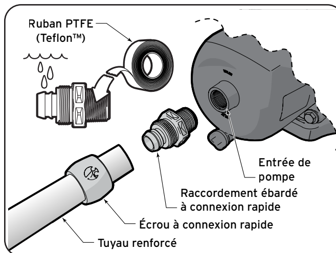
Figure 9. Installation à connexion rapide
